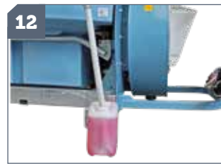
12 IT: Incorporatore aspirante di prodotti a tubo / EN: Sucking device for powders with pipe / FR: Incorporateur de poudre avec tuyau / DE: Spritzmittel-Einfüllschleuse mit Schlauch / ES: Incorporador aspirante de productos con caño
